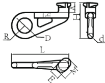
SLR633 G80 GANCHO IZQUIERDO CONTENEDOR
