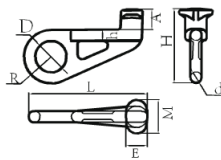
SLR633 G80 GANCHO CONTENEDOR
